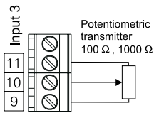
h) Auxiliary potentiometric input
