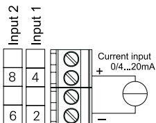
e) Current input
